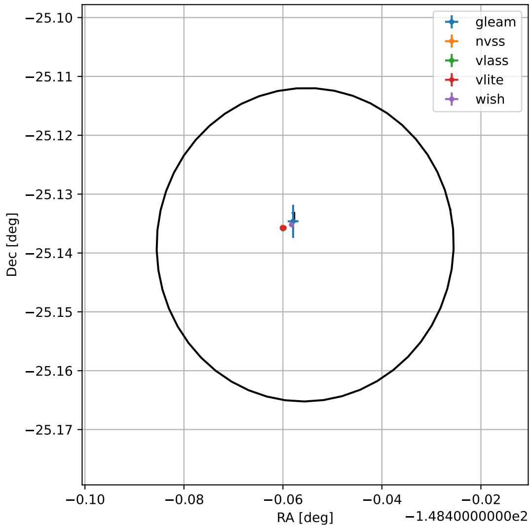
4FGL J1406.1-2508
