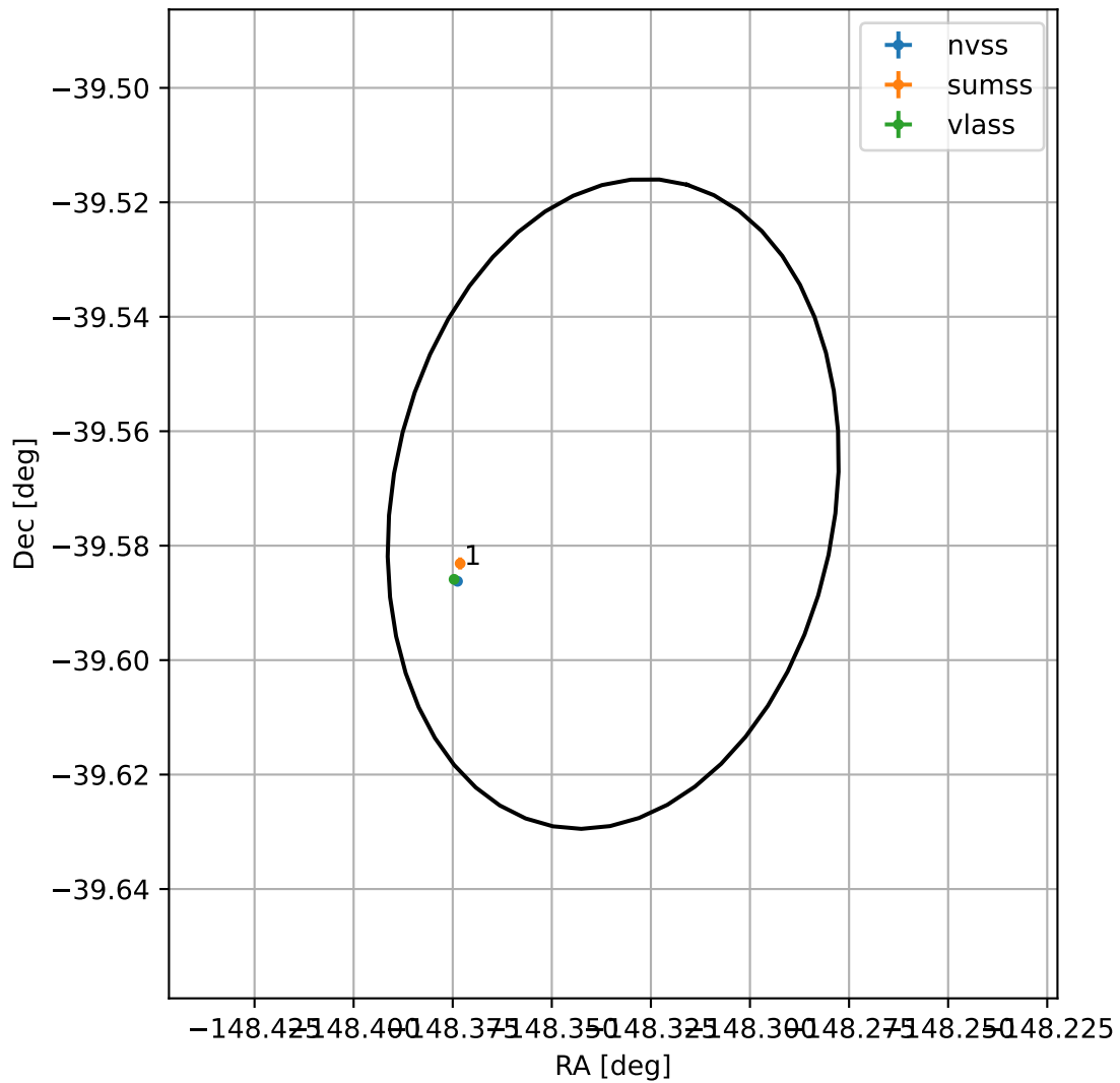
4FGL J1406.6-3934
