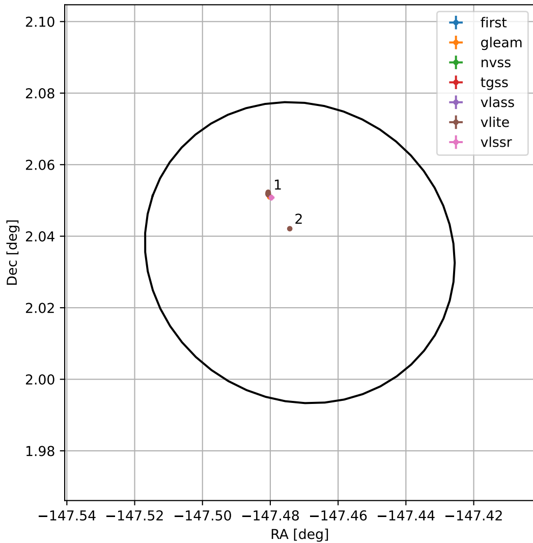
4FGL J1410.1+0202
