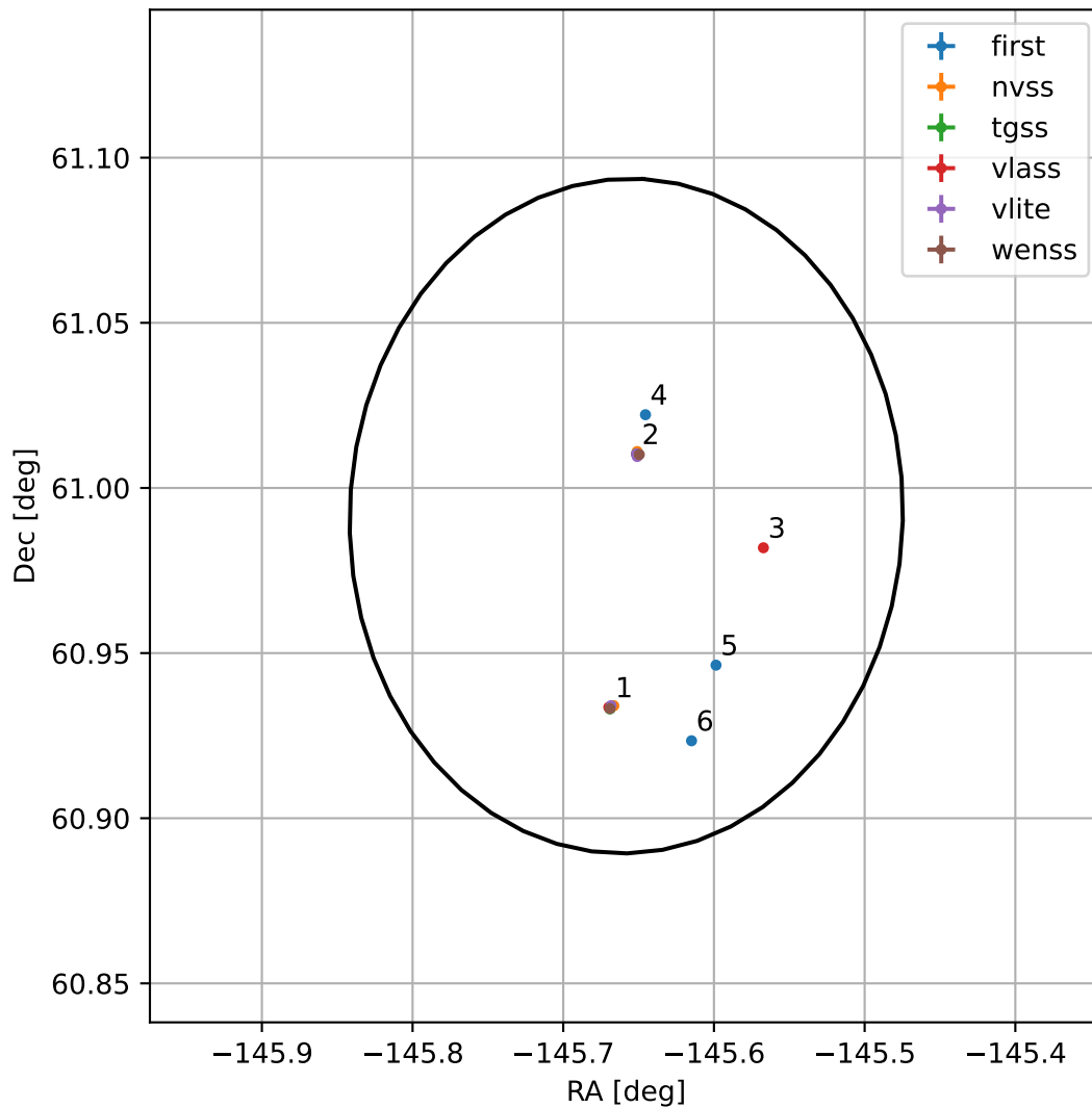
4FGL J1417.3+6059
