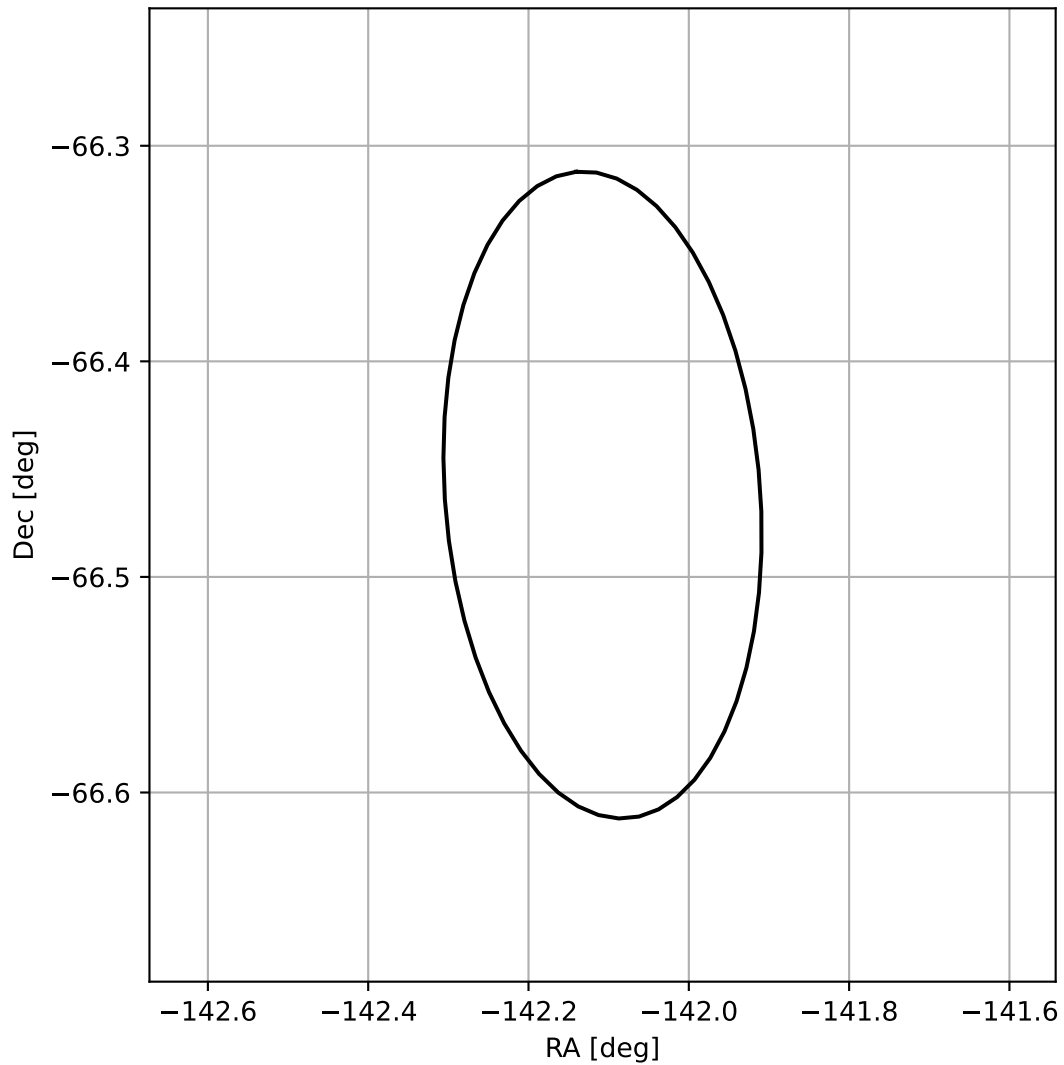
4FGL J1431.5-6627
