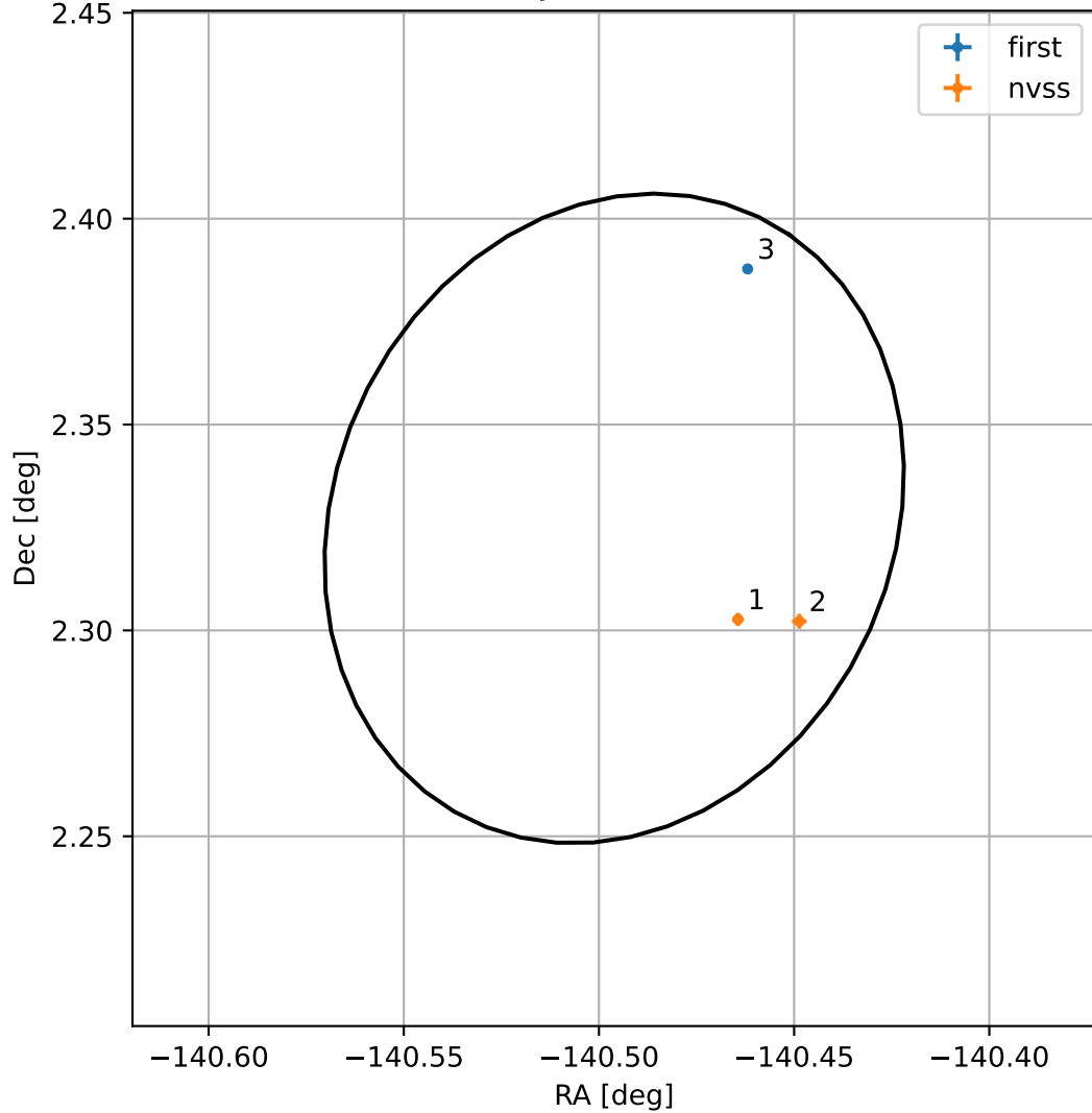
4FGL J1438.0+0219
