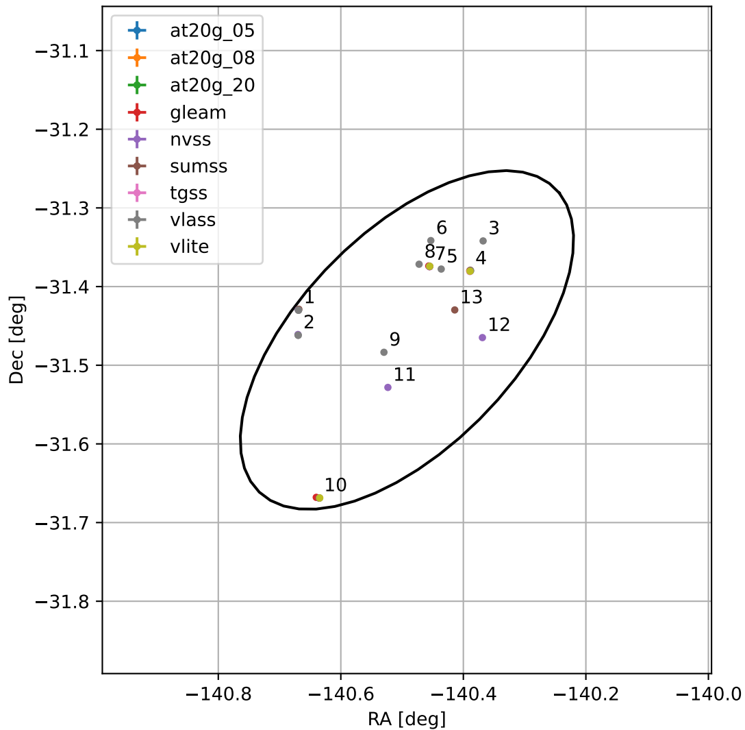
4FGL J1438.0-3128
