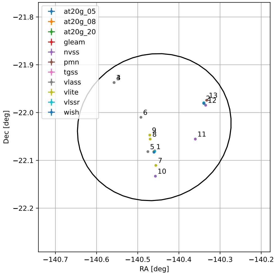
4FGL J1438.1-2201
