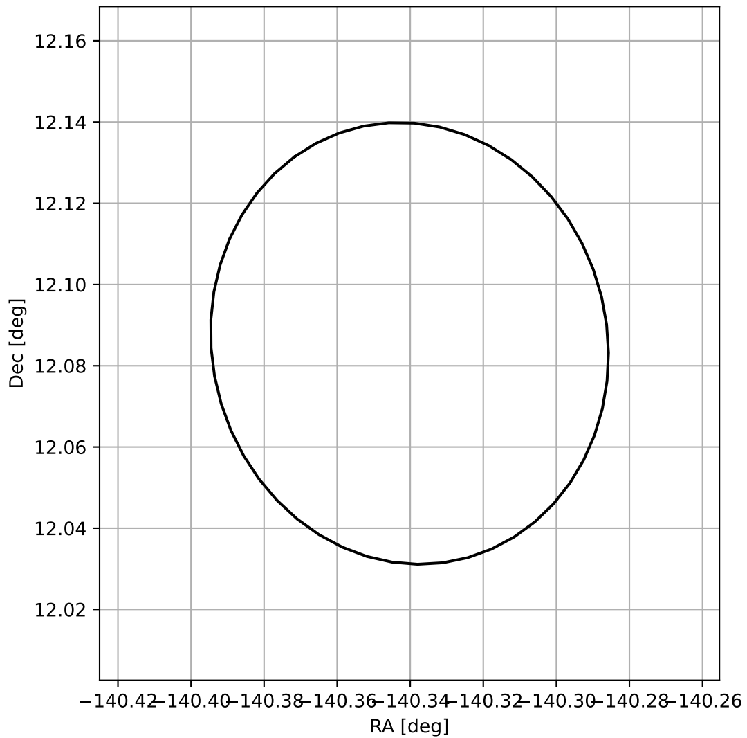
4FGL J1438.6+1205
