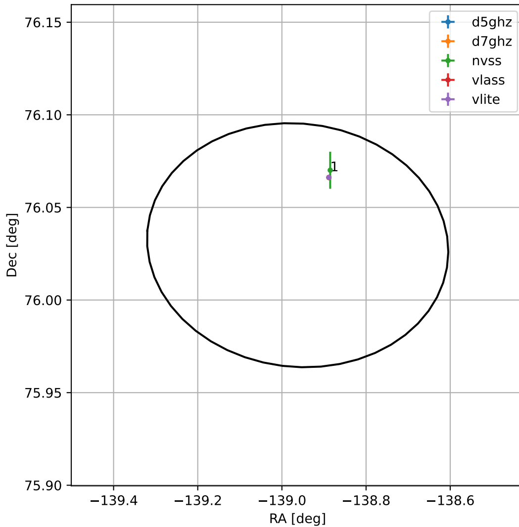
4FGL J1444.1+7601
