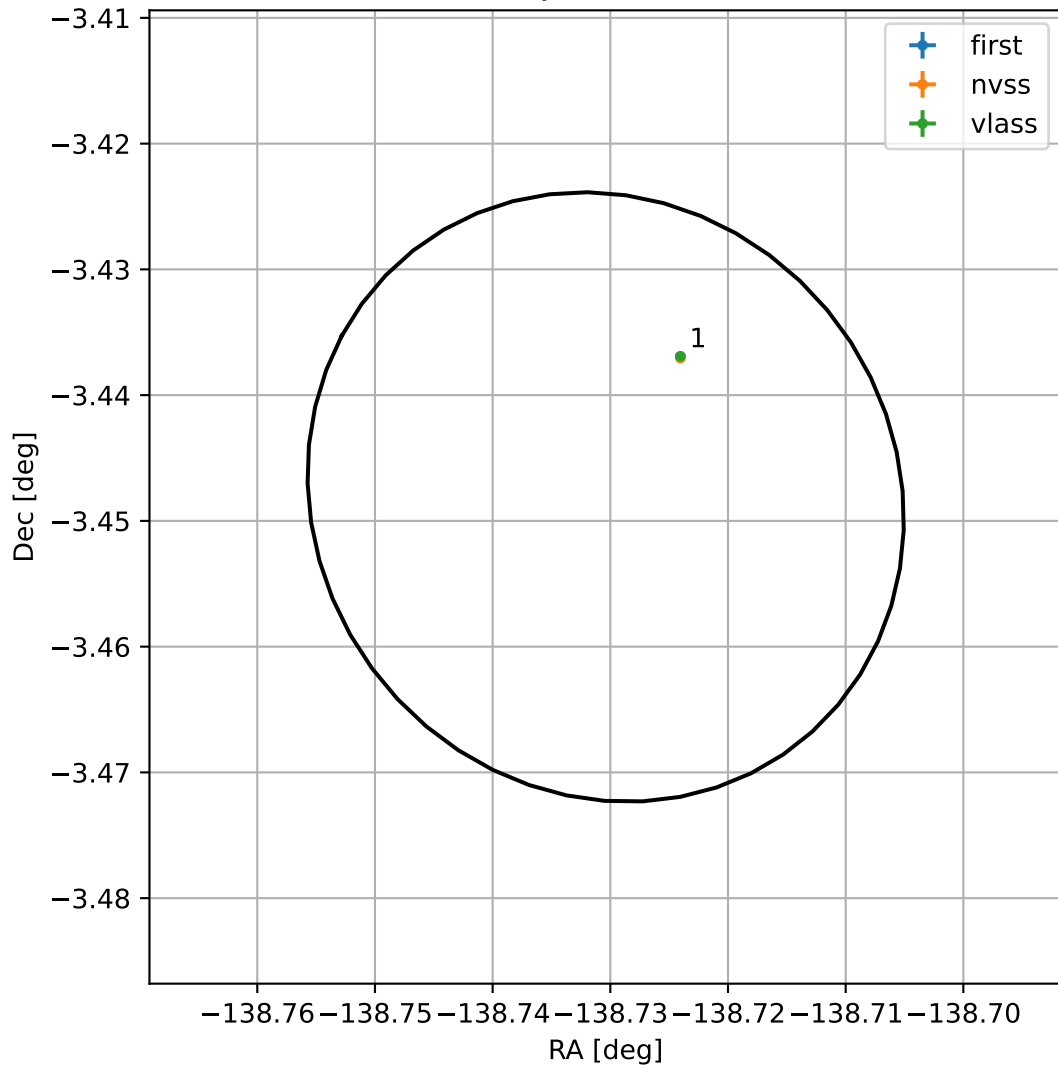
4FGL J1445.0-0326
