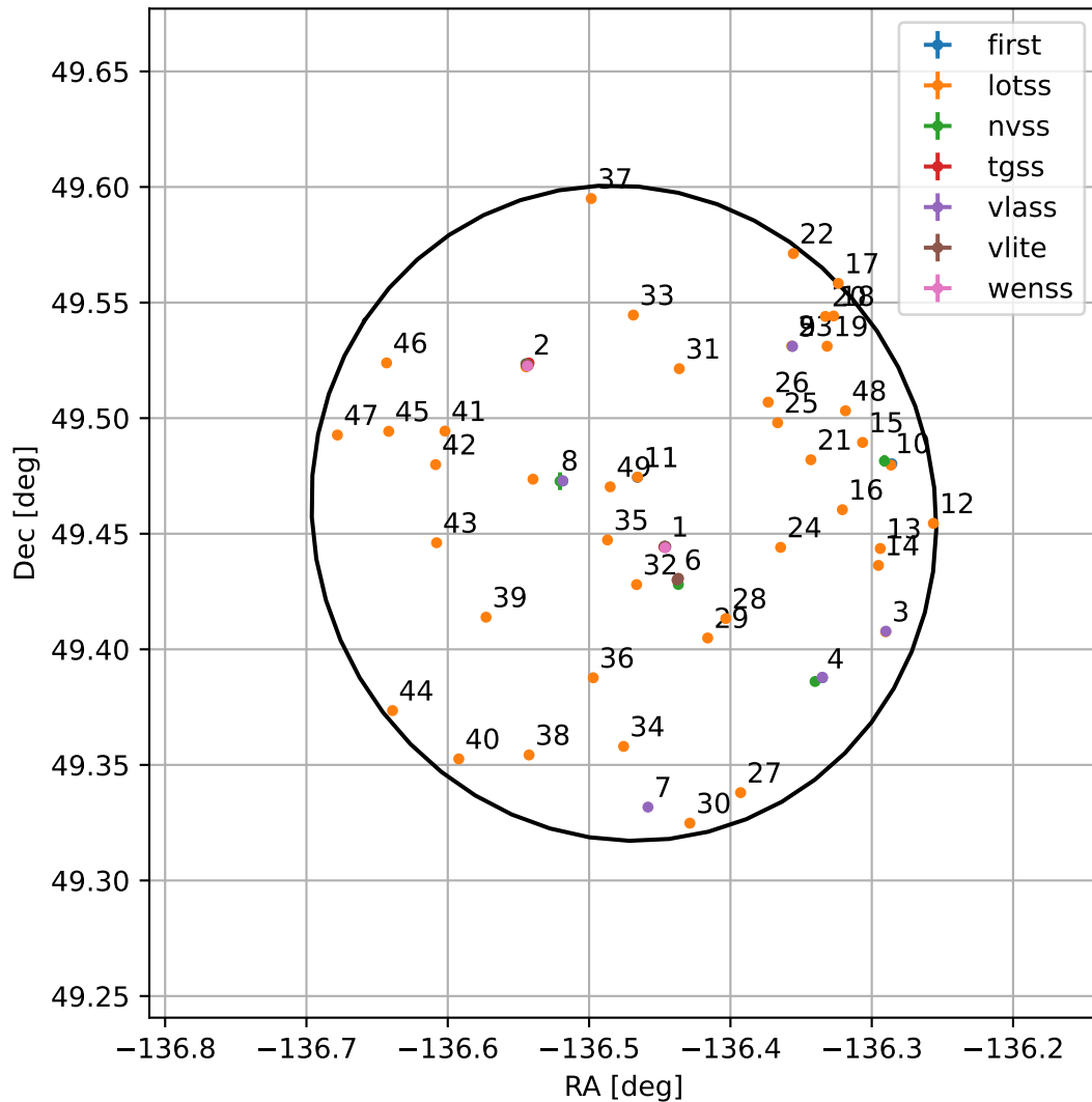
4FGL J1454.0+4927
