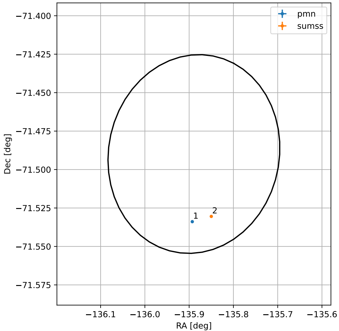
4FGL J1456.4-7129
