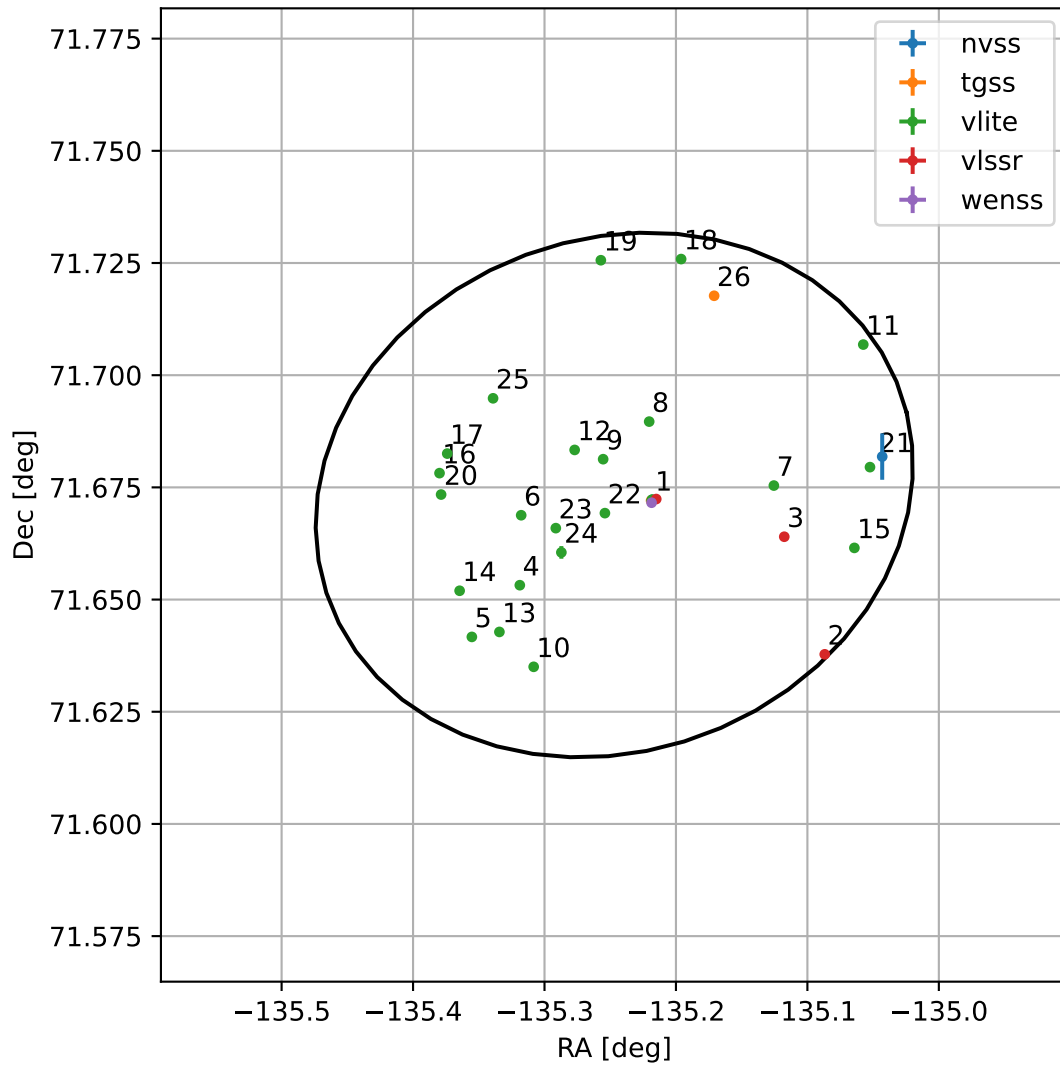
4FGL J1459.0+7140
