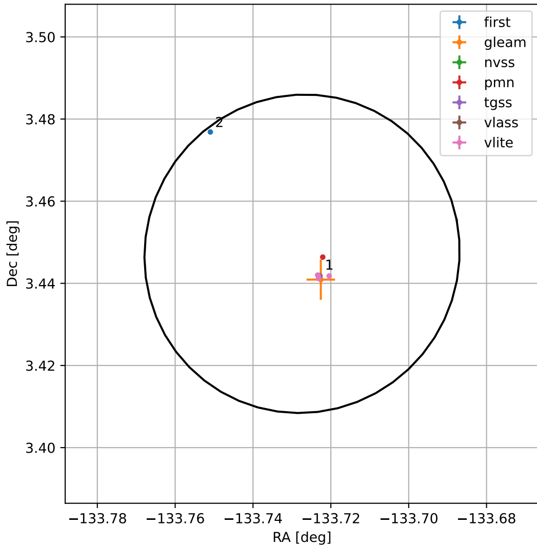
4FGL J1505.0+0326
