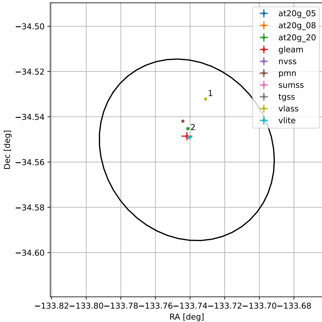
4FGL J1505.0-3433
