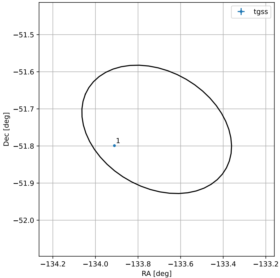
4FGL J1505.1-5145
