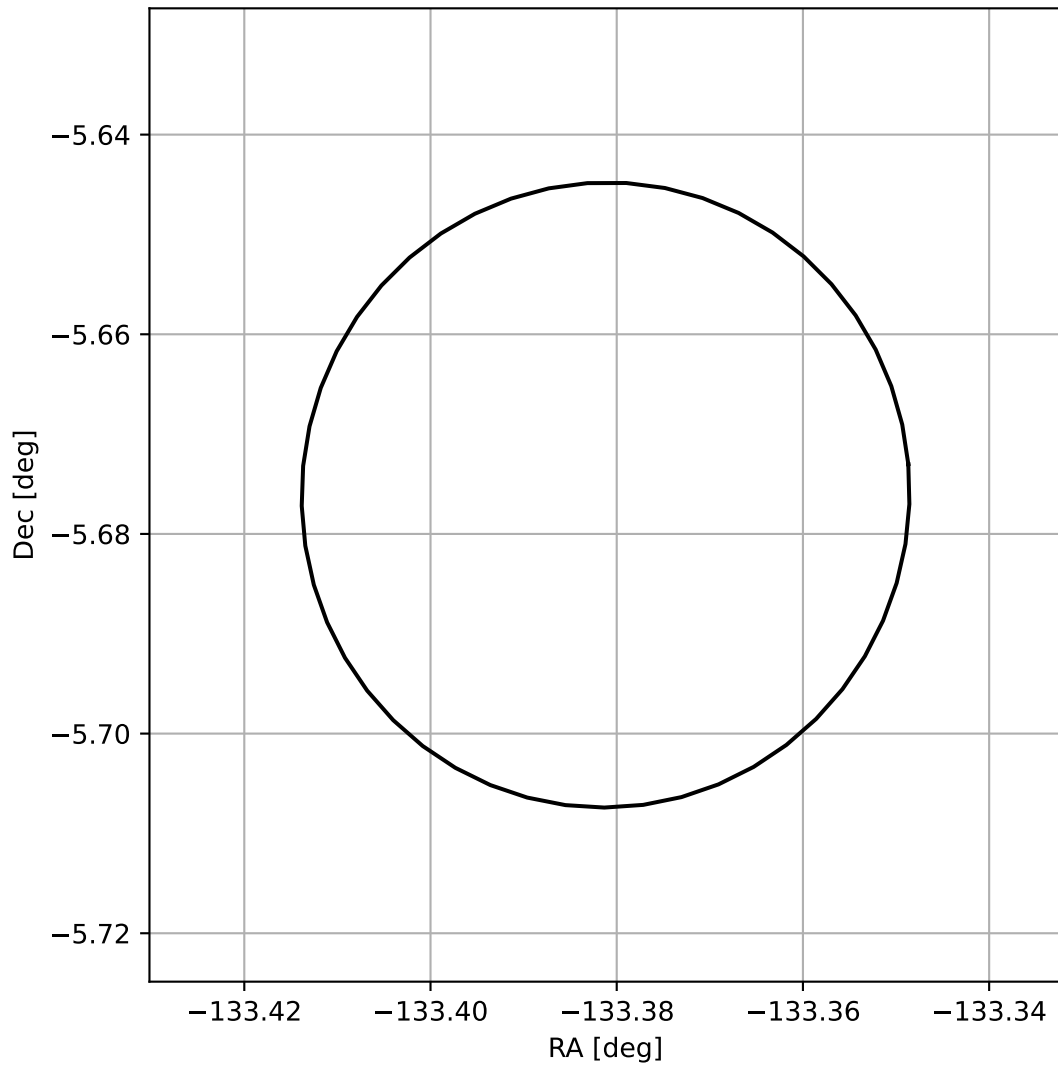
4FGL J1506.4-0540
