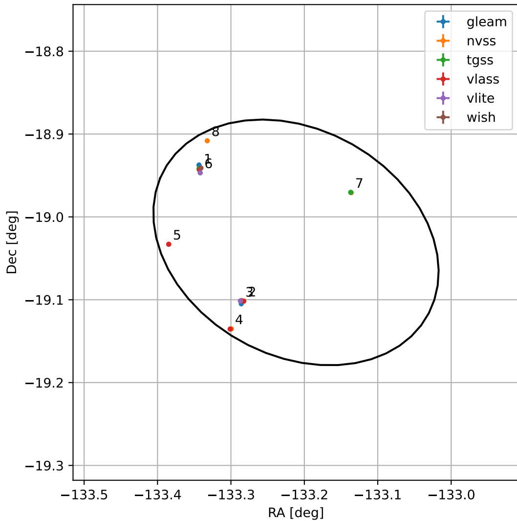
4FGL J1507.1-1901
