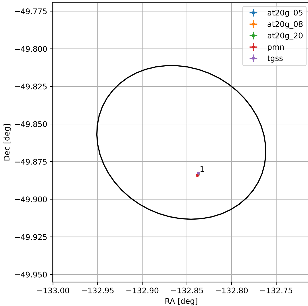
4FGL J1508.5-4951
