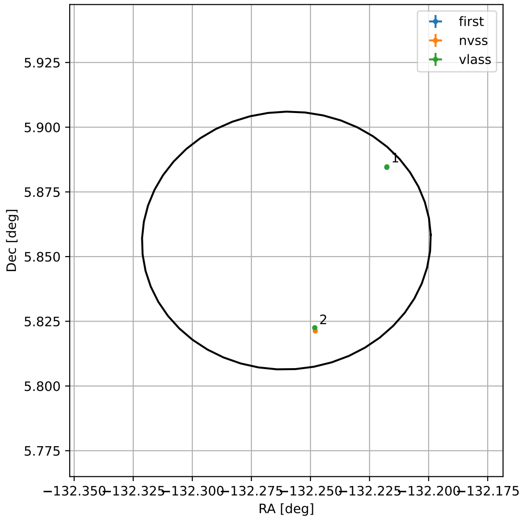
4FGL J1510.9+0551
