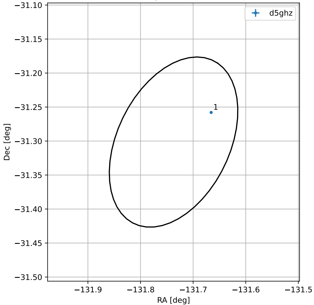
4FGL J1513.0-3118
