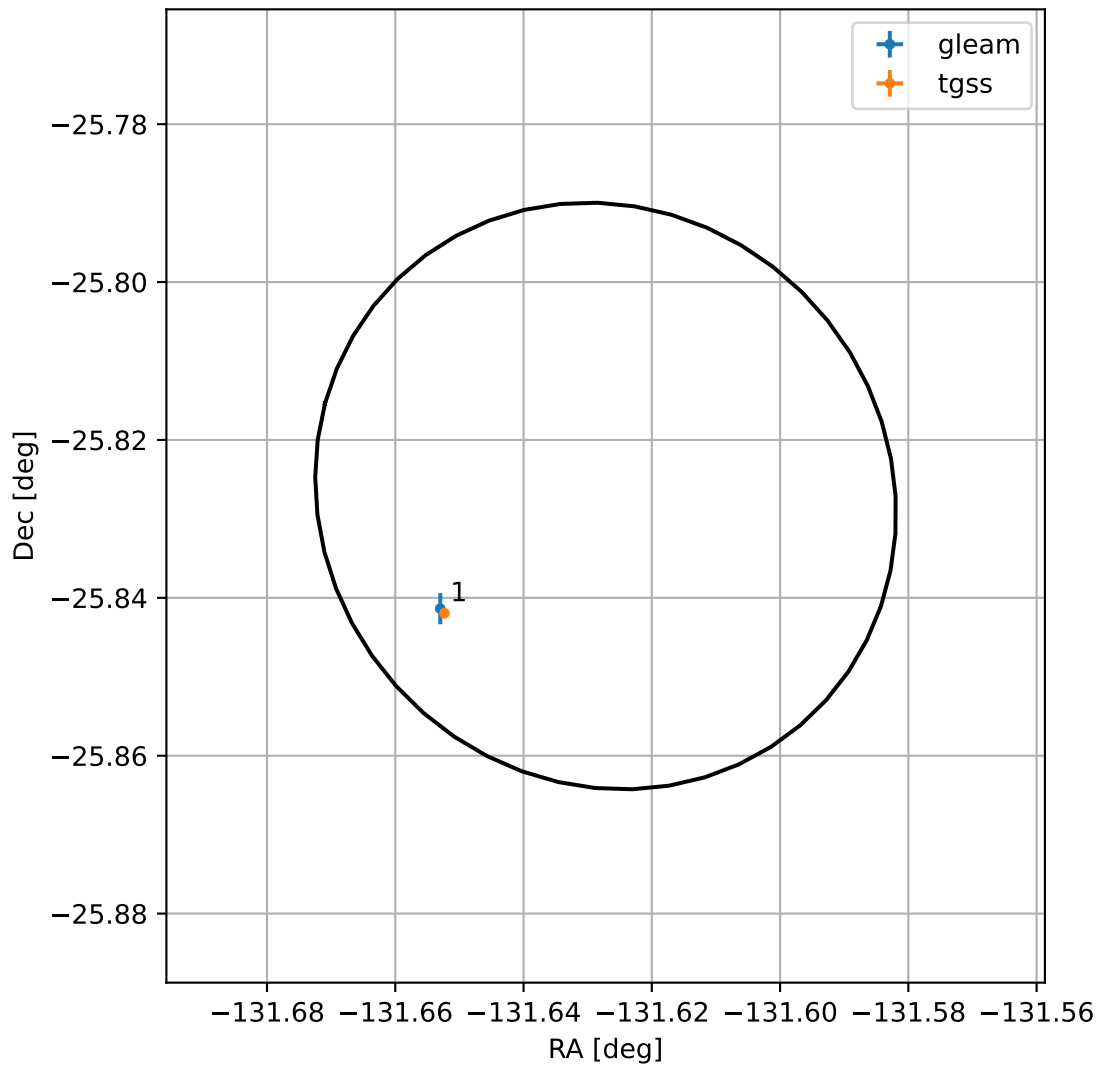
4FGL J1513.4-2549
