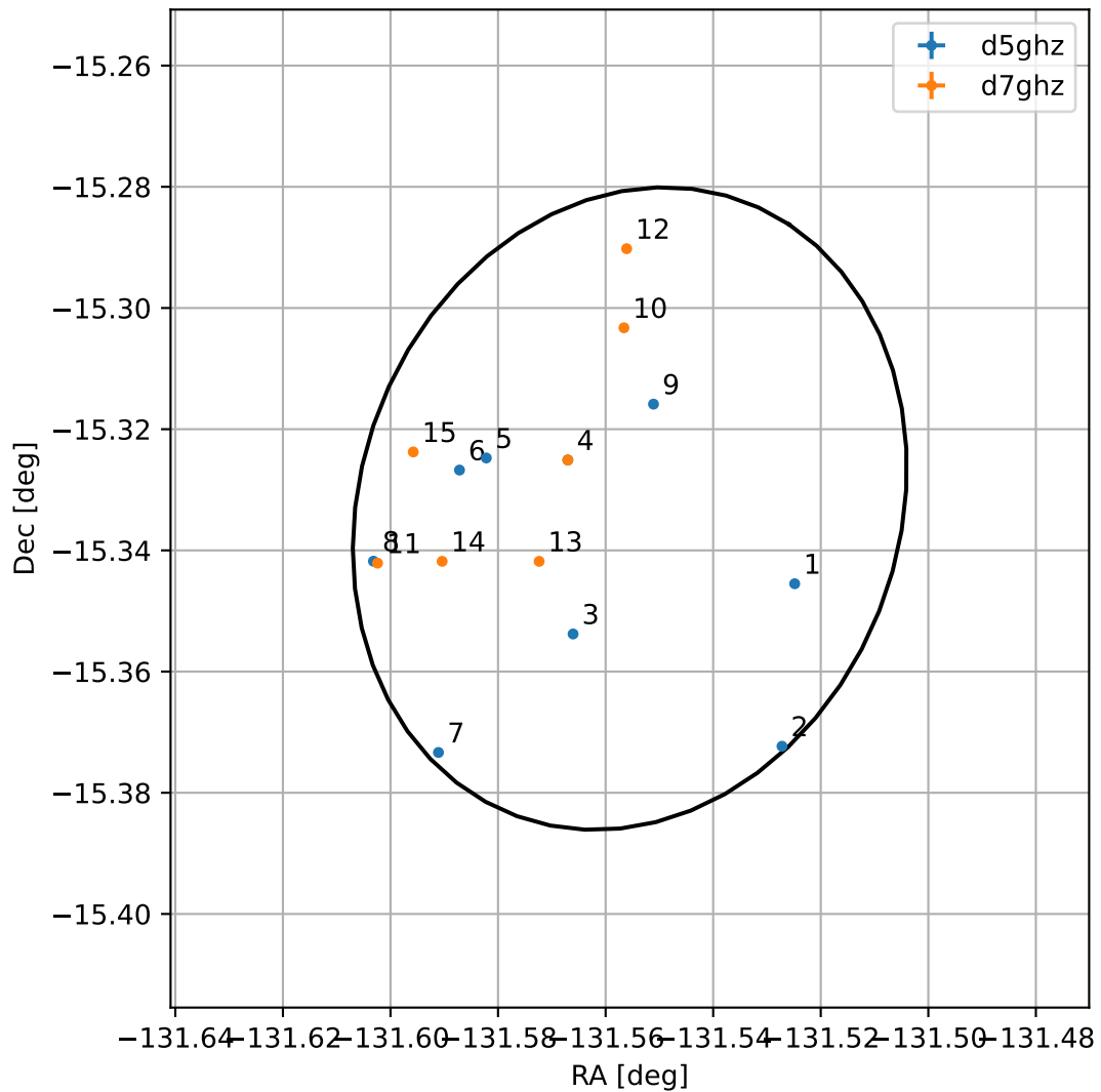
4FGL J1513.7-1519
