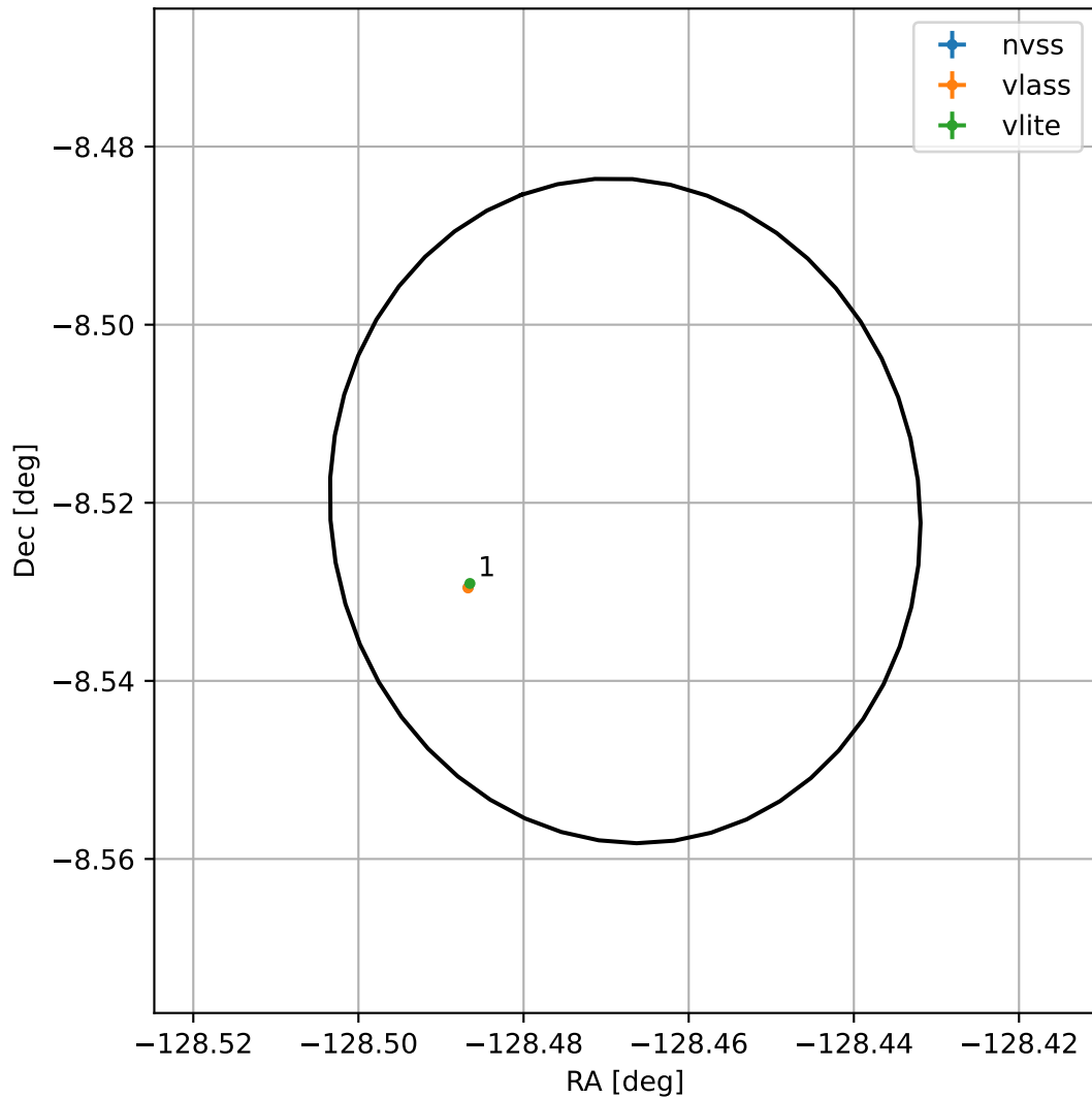
4FGL J1526.1-0831
