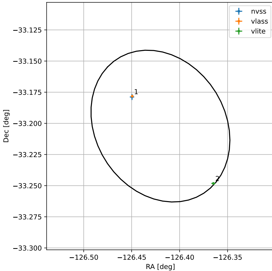
4FGL J1534.3-3312
