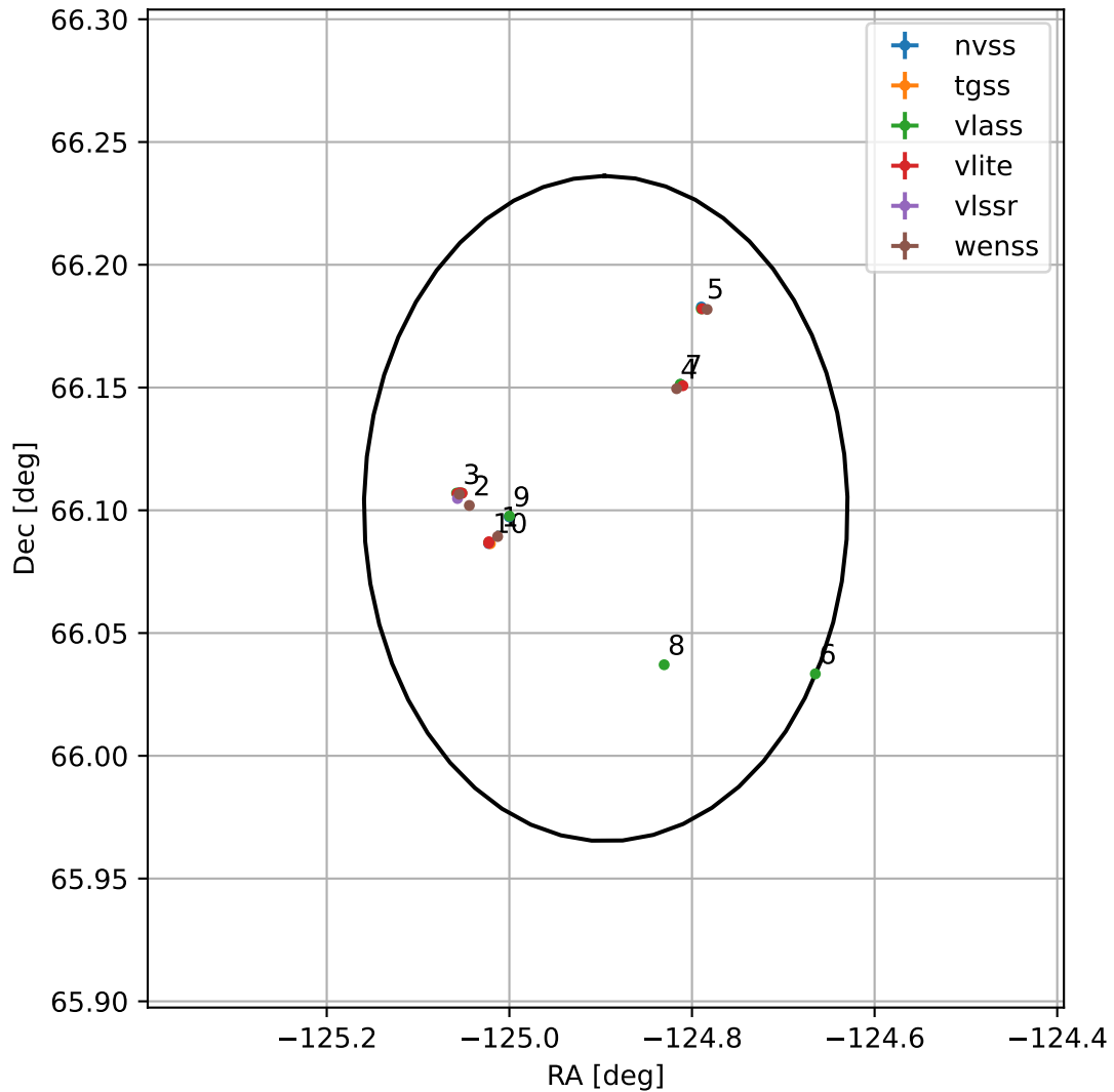
4FGL J1540.4+6606
