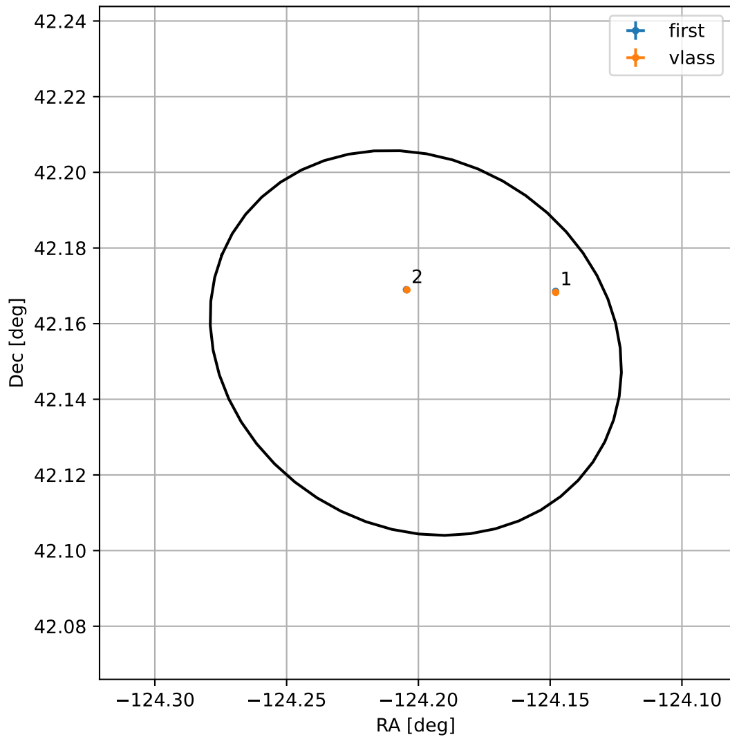
4FGL J1543.1+4209
