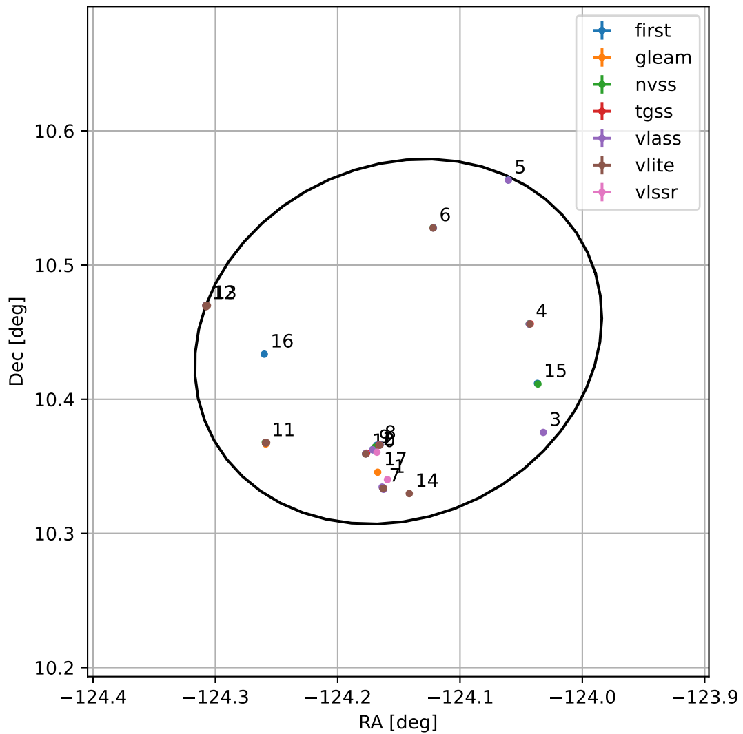
4FGL J1543.3+1026
