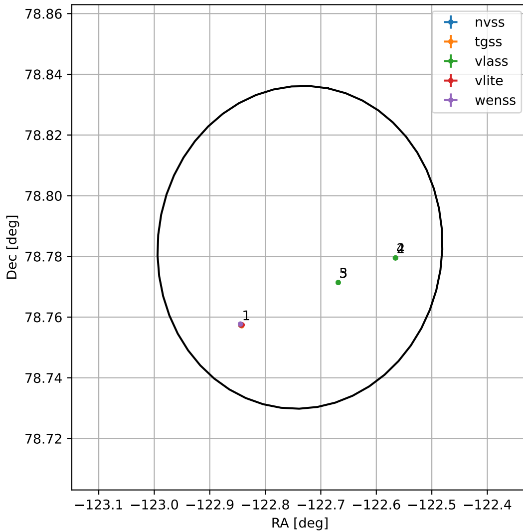
4FGL J1549.0+7846
