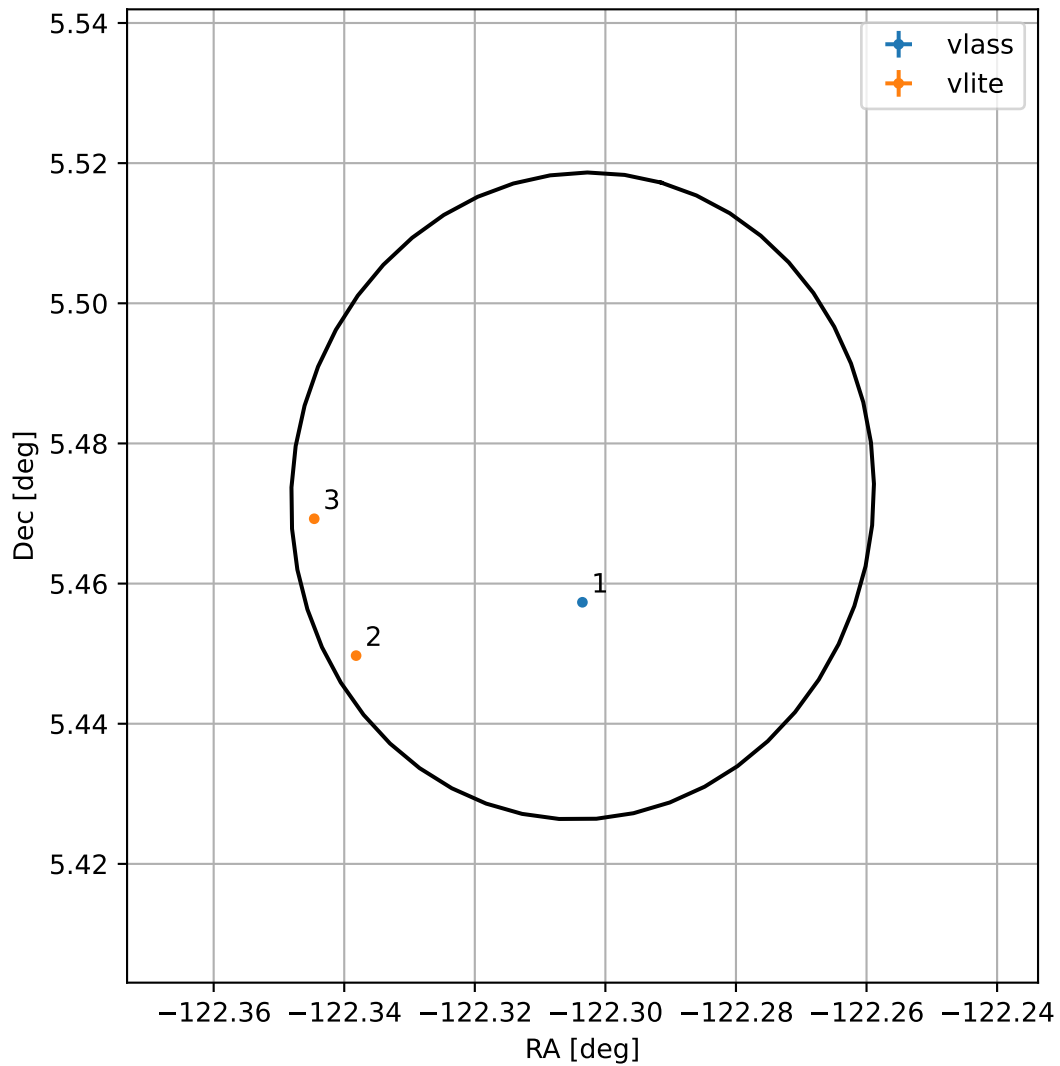
4FGL J1550.7+0528
