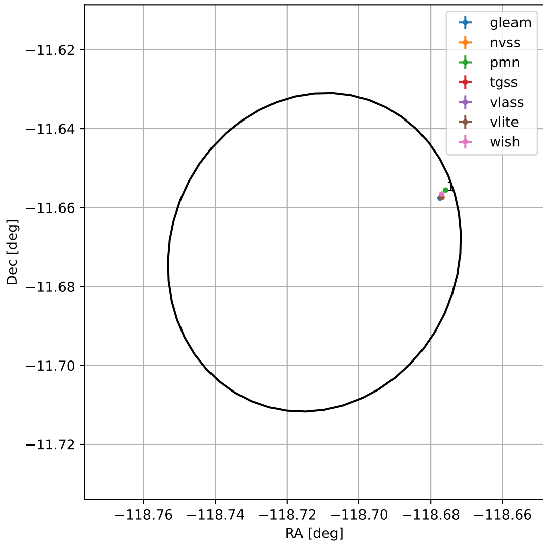
4FGL J1605.1-1140
