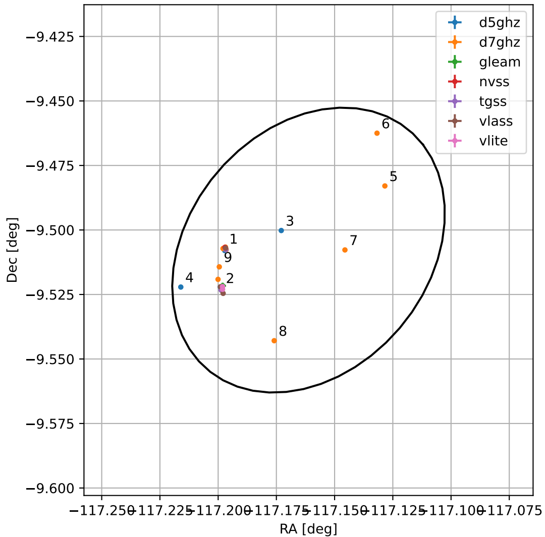
4FGL J1611.3-0930
