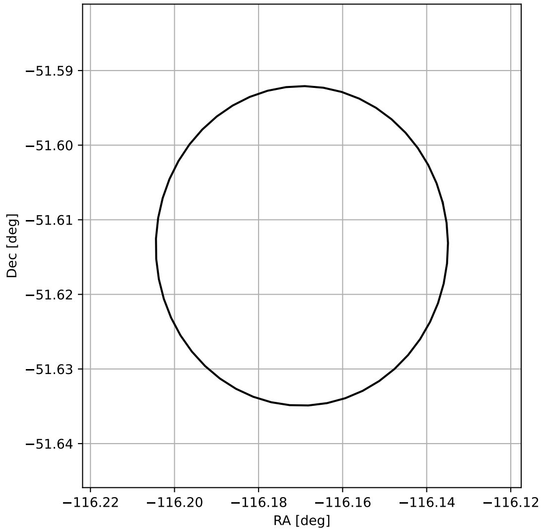
4FGL J1615.3-5136
