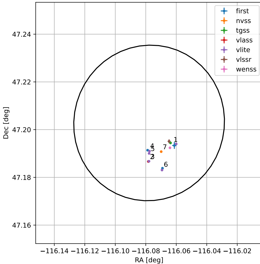
4FGL J1615.6+4712
