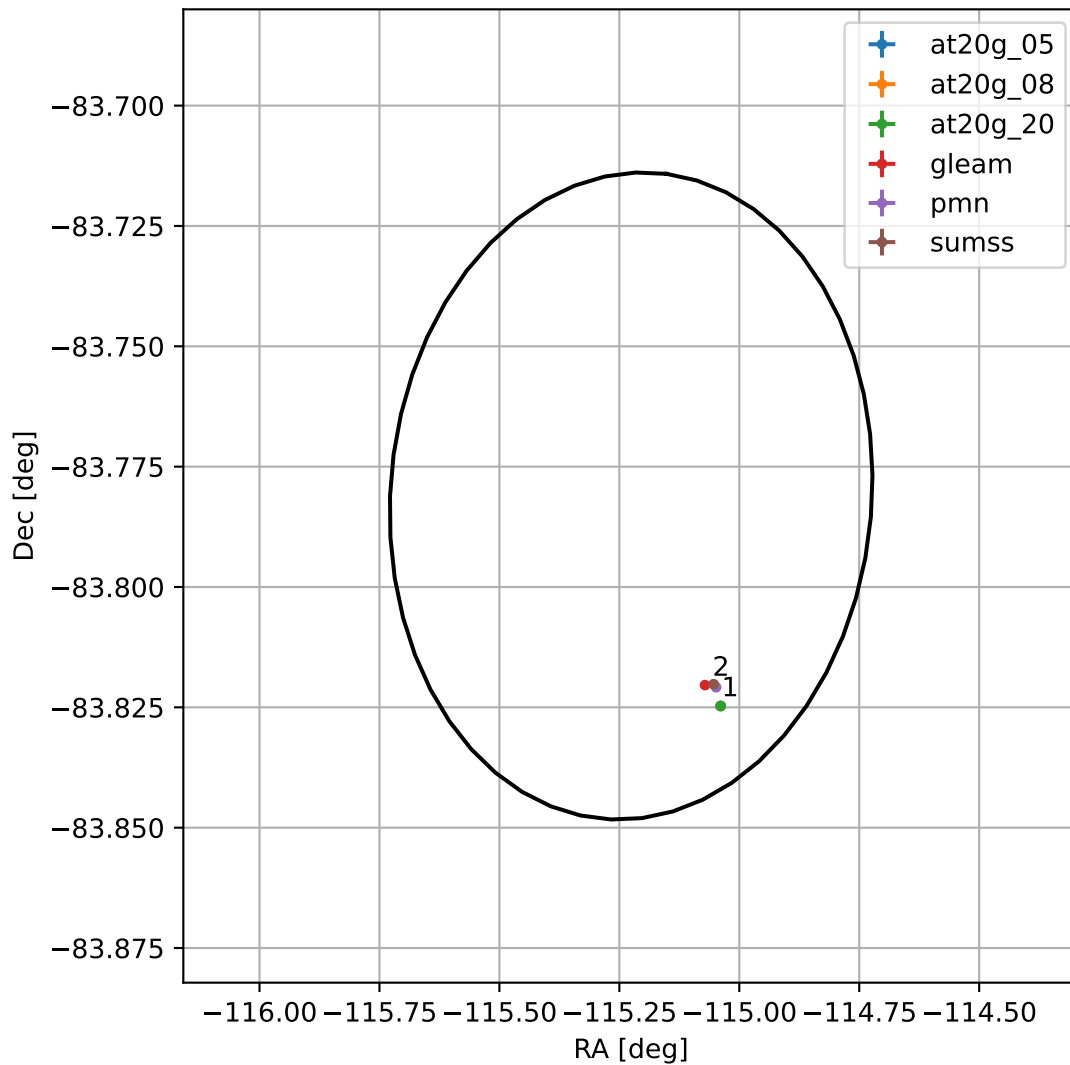
4FGL J1619.0-8346
