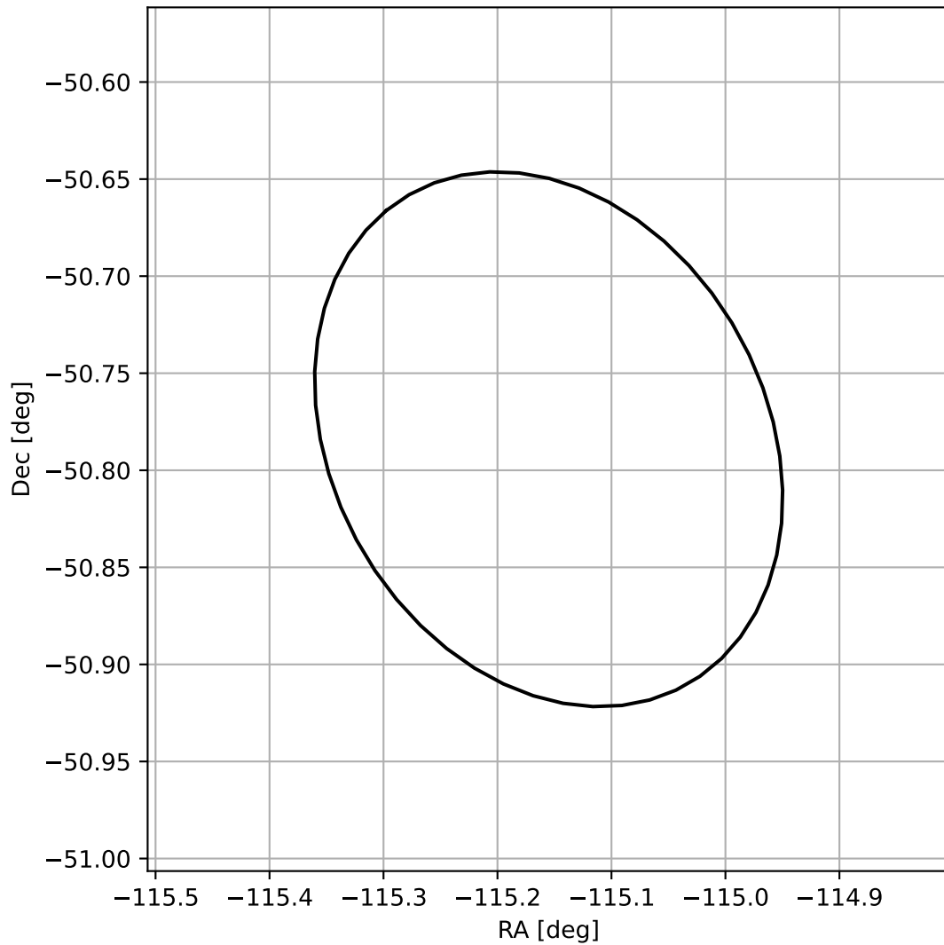
4FGL J1619.3-5047
