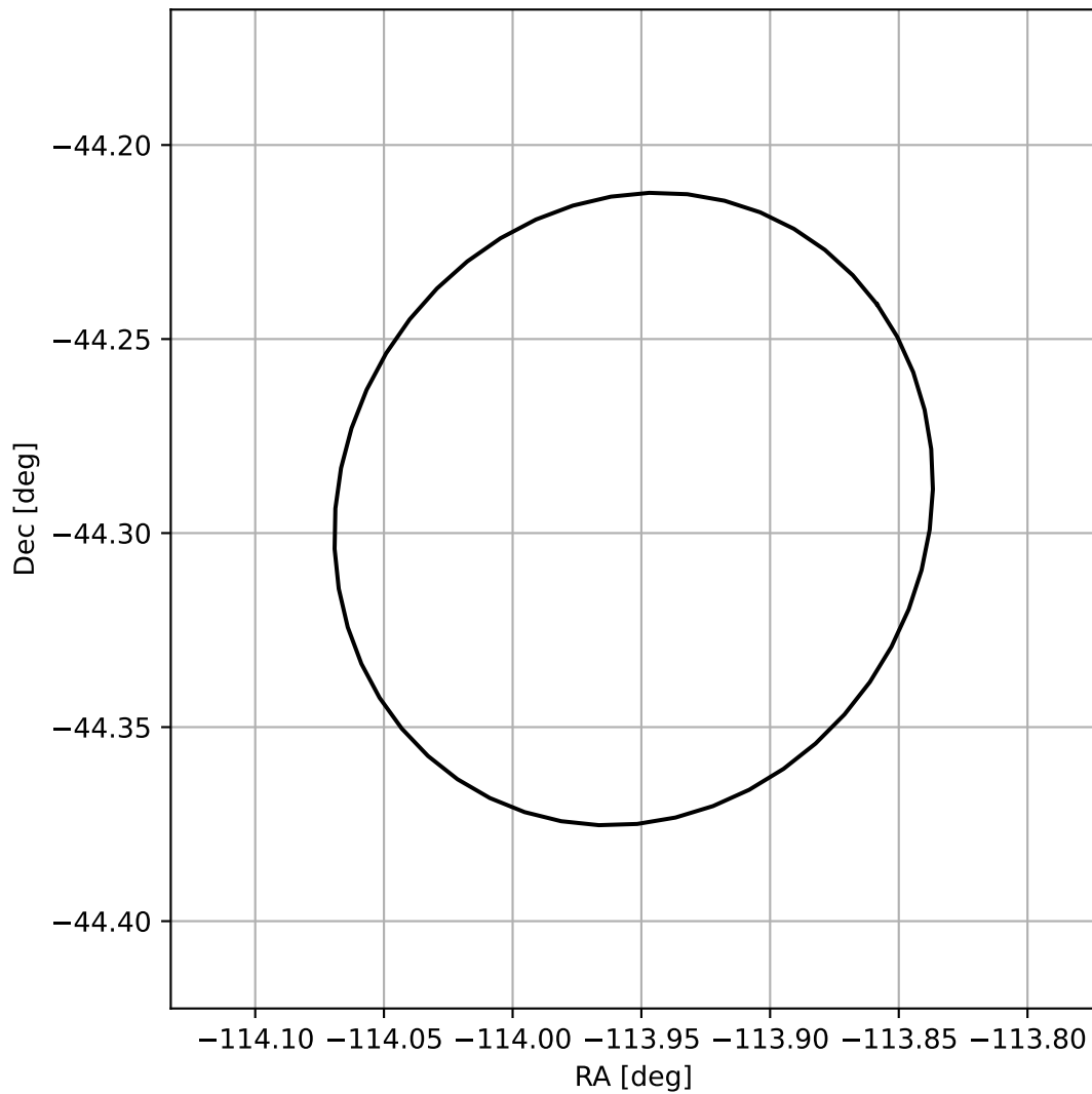
4FGL J1624.1-4417
