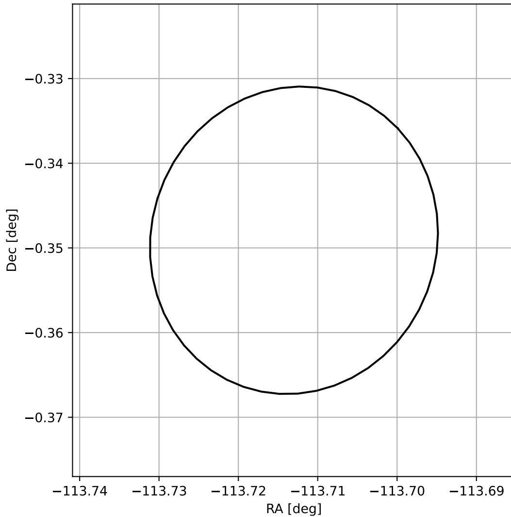
4FGL J1625.1-0020
