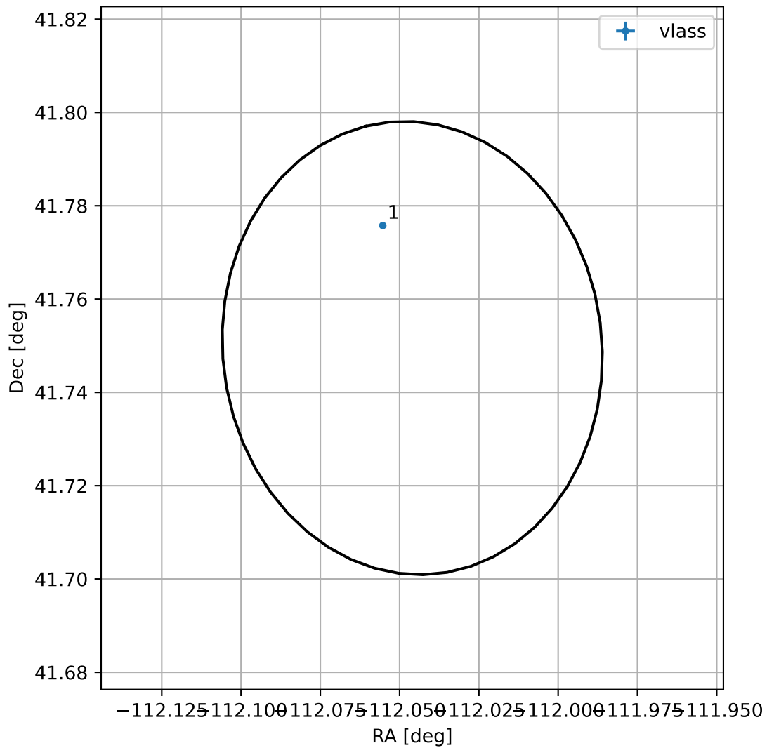
4FGL J1631.8+4144
