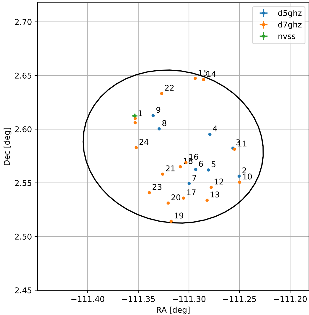
4FGL J1634.7+0235
