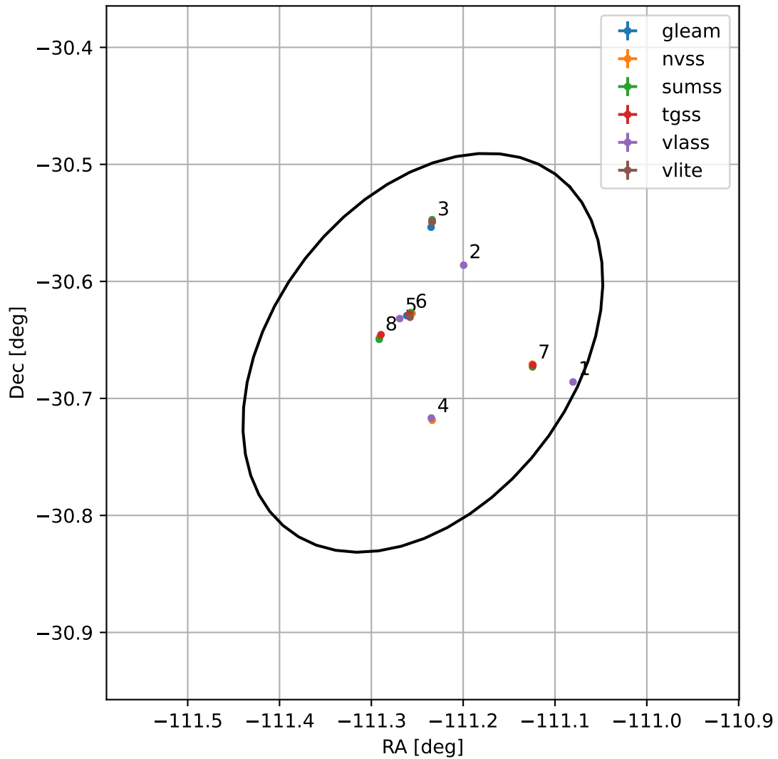
4FGL J1635.0-3039
