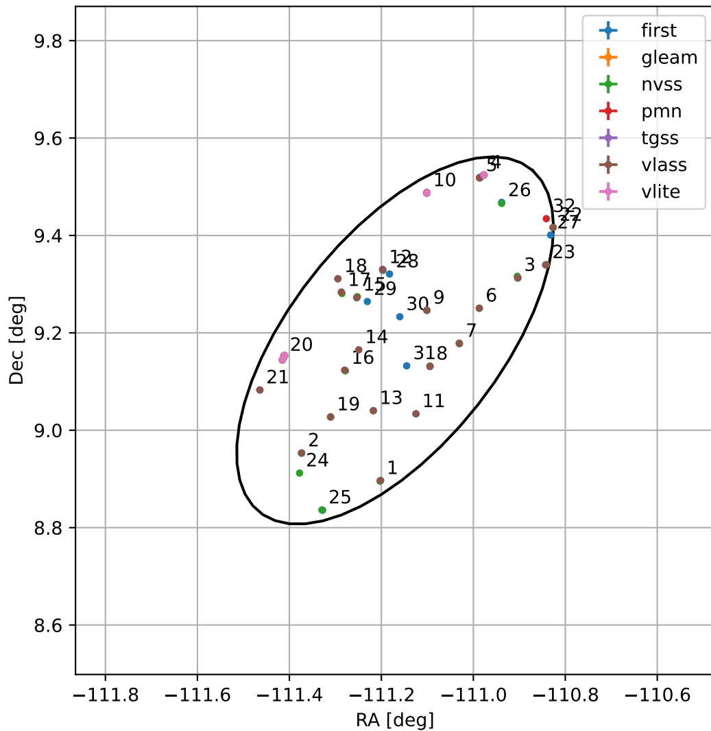
4FGL J1635.3+0911
