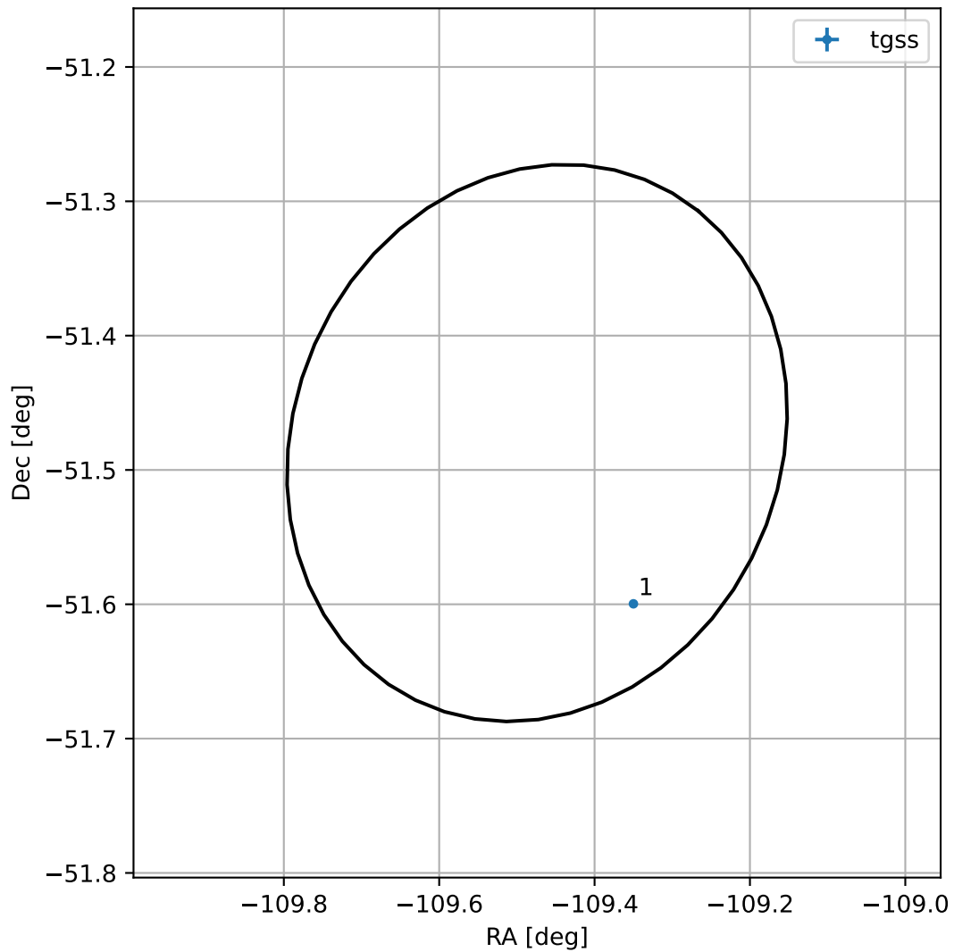
4FGL J1642.1-5128
