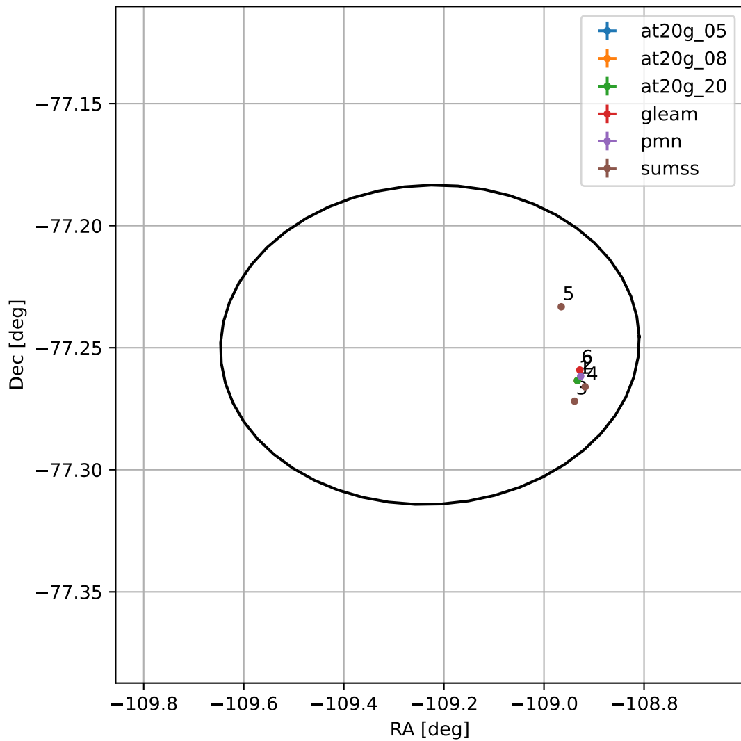
4FGL J1643.0-7714
