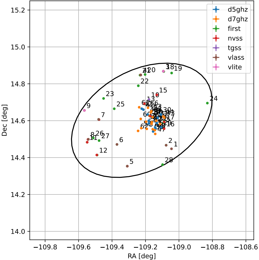
4FGL J1643.1+1436
