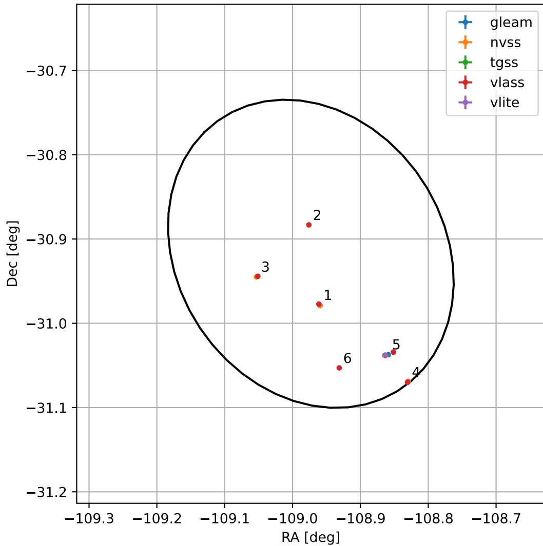
4FGL J1644.1-3055
