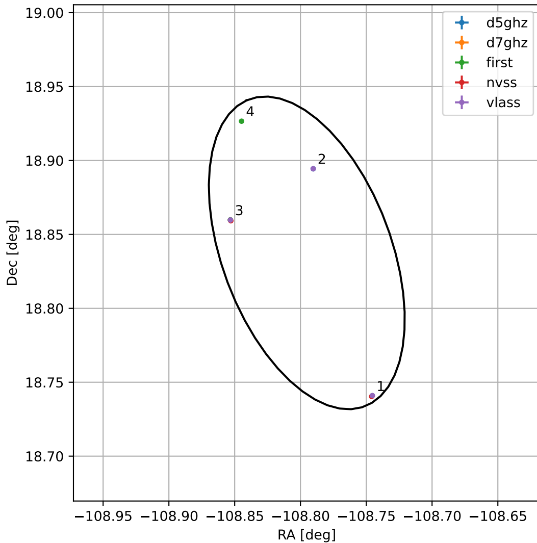
4FGL J1644.8+1850
