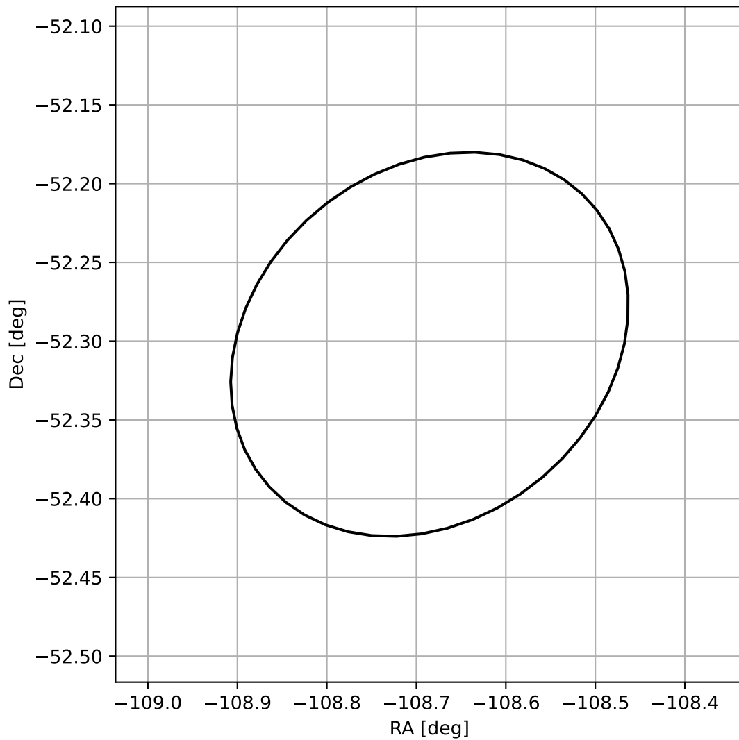
4FGL J1645.2-5218
