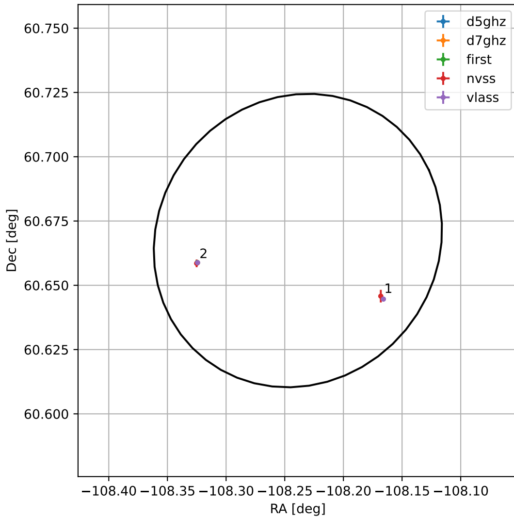
4FGL J1647.0+6040
